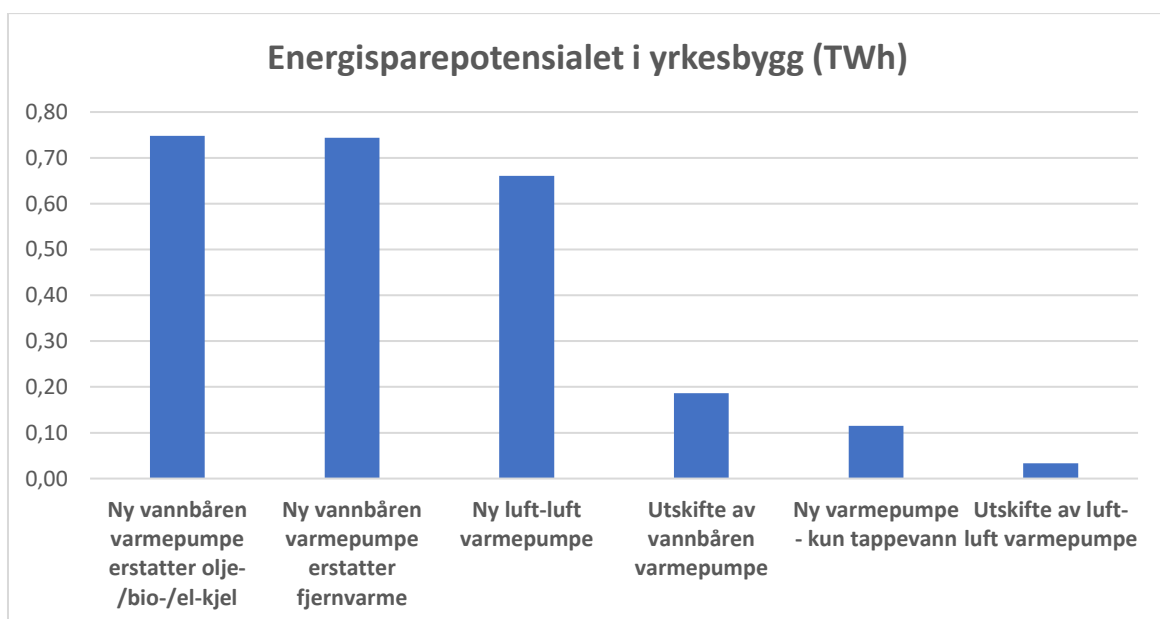
Figur 2: Energisparepotensialet ved installasjon/utskifte av varmepumper i eksisterende yrkesbygg
